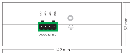
后面板视图
