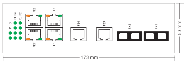
后面板视图
