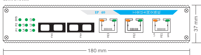
前面板视图
