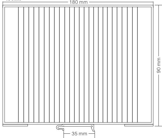
俯视图
