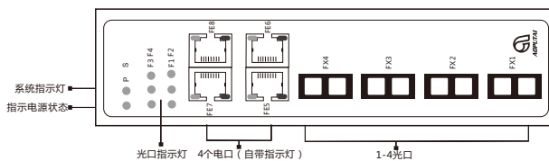
侧面板视图
