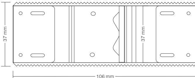
后面板视图
