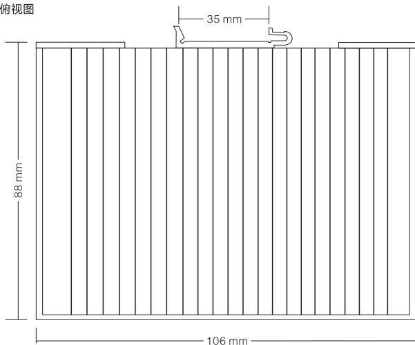
俯视图
