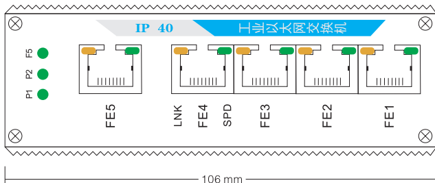
前面板视图
