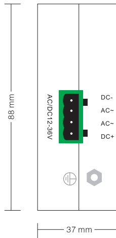
侧面板视图
