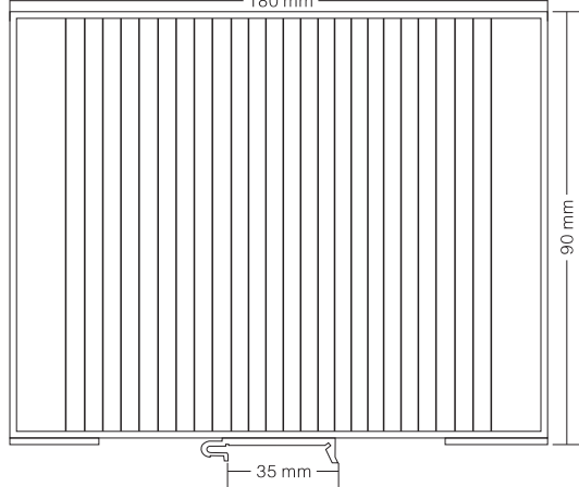
俯视图
