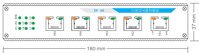
前面板视图
