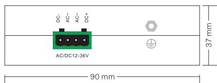
侧面板视图
