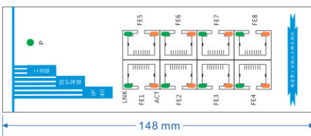
前面板视图
