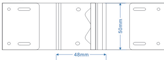
后面板视图
