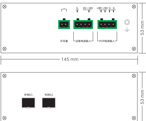
侧面板视图
