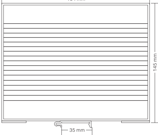
俯视图
