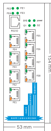
前面板视图
