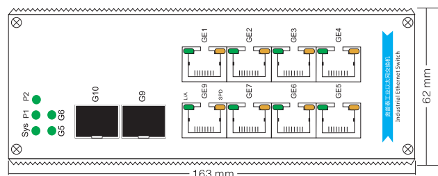
侧面板视图
