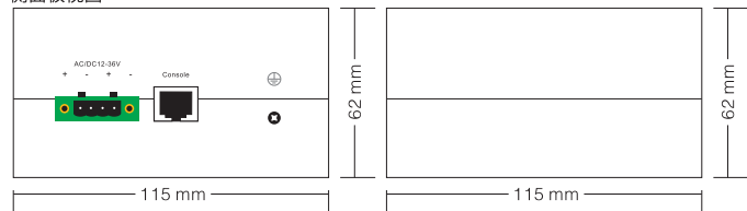
侧面板视图
