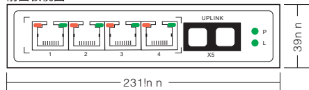
后面板视图
