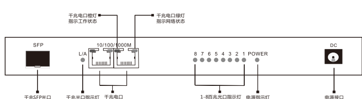
后面板视图
