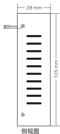
侧视图
